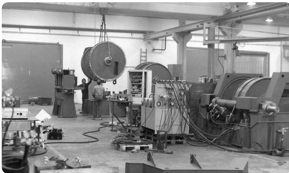
Spillene til Jugoslavien i montagehallen. Forrest et Inline spil under funktionstest og bagerst et Waterfall under montage.
